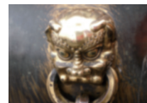
MPEG4
